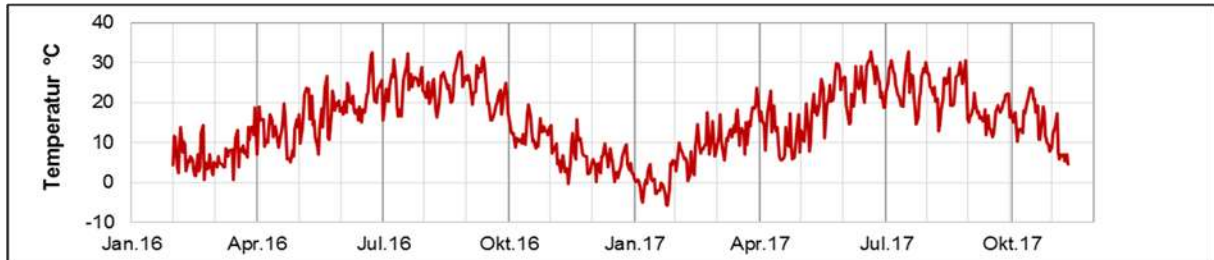
Abbildung 15: Ganglinie der Temperatur um 14 Uhr der Klimastation Stuttgart-Flughafen
